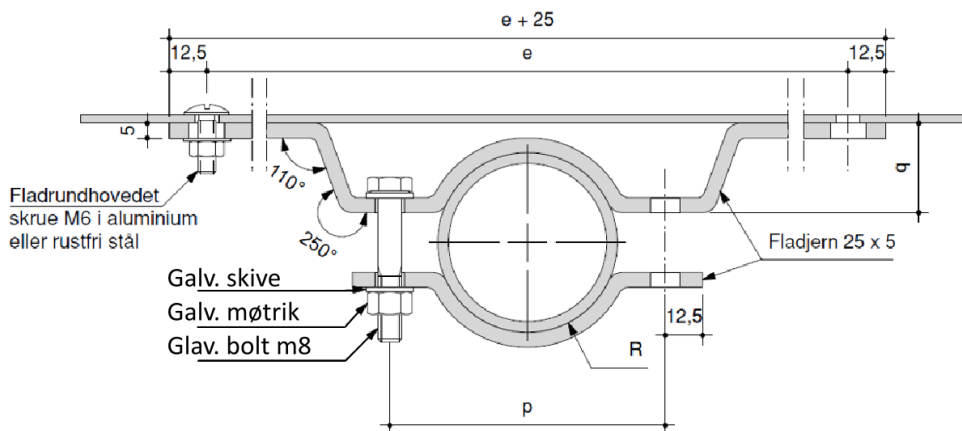
Snit A-A 1:2
